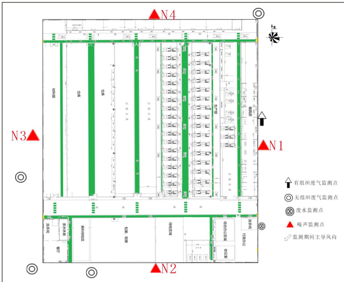
图 3.1-2 厂区平面布置图
